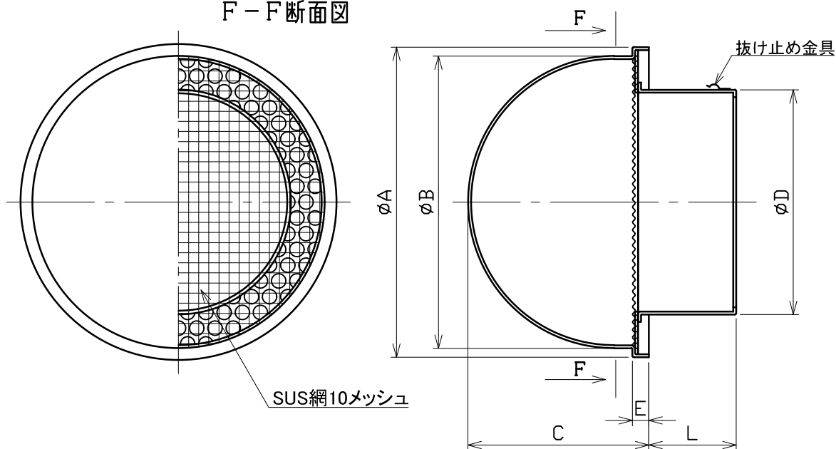
F-F断面図
