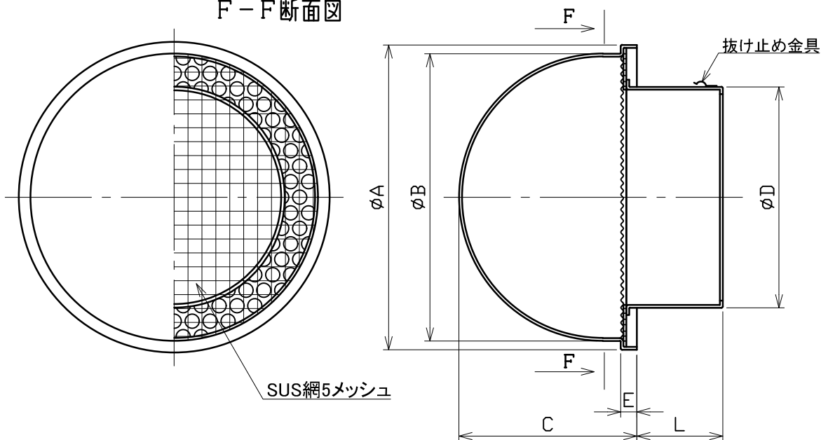
F-F断面図
