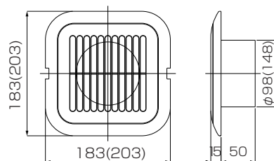
《 本体構造説明図 》 ※( )内はφ150寸法
