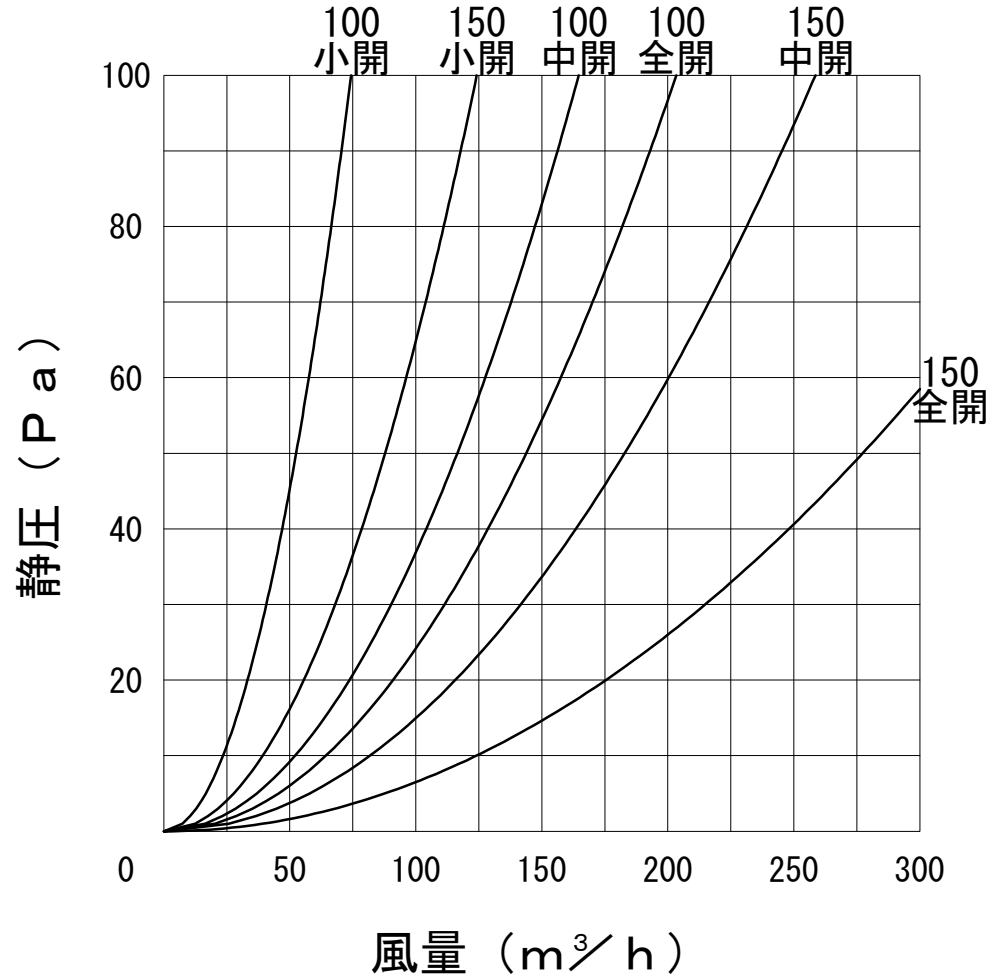
圧力損失曲線図 (給気)
