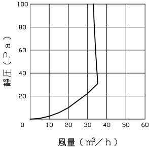
■ 圧力損失曲線図 (給気)
