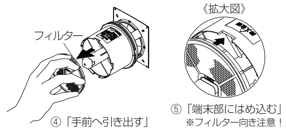
④「手前へ引き出す」
