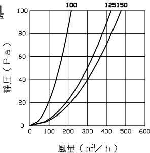
■圧力損失曲線図（給気）
