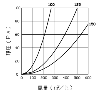
■ 压力损失曲线图（排气）
