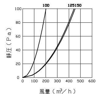
■ 压力损失曲线图（排气）
