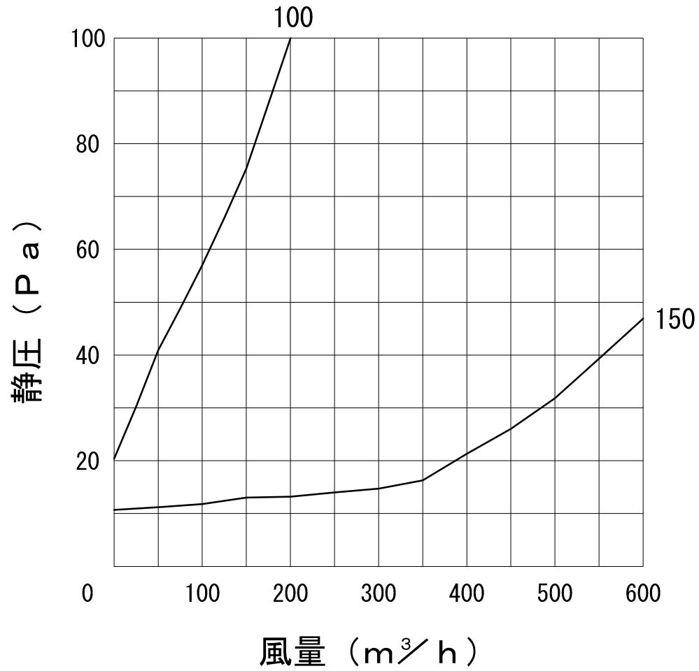
圧力損失曲線図
